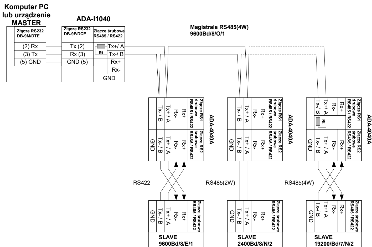
Rys 6. Przykładowe podłączenie ADA-4040A do magistrali RS485(2W) 2-przewodowej oraz separacja galwaniczna urządzeń SLAVE
