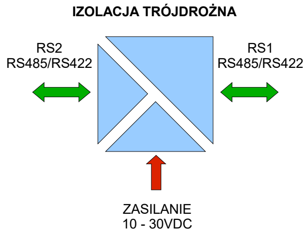
Rys 2. Struktura izolacji
